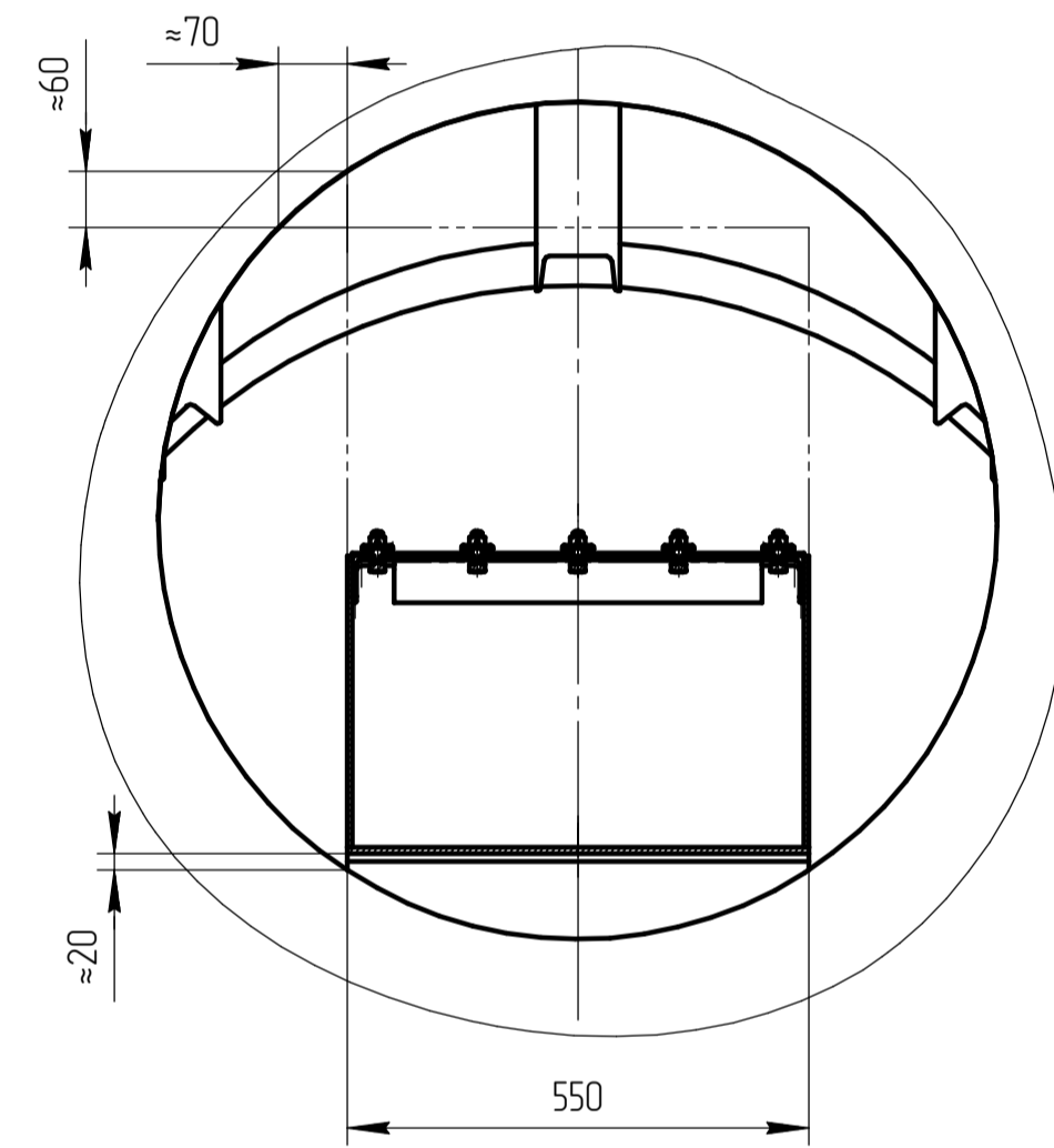
Л-Л(8В)
