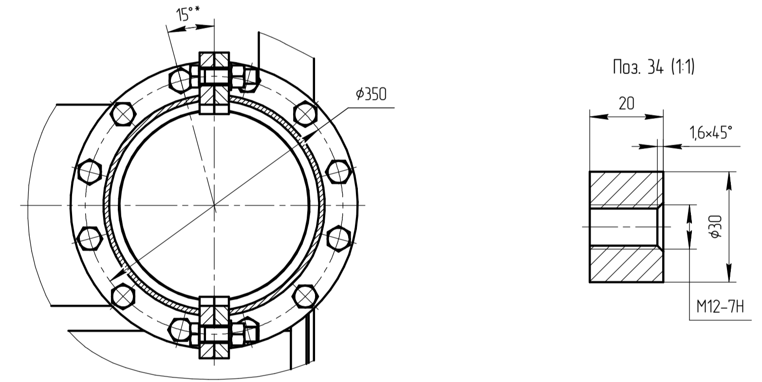
Д-Д(1:5)(7В)
