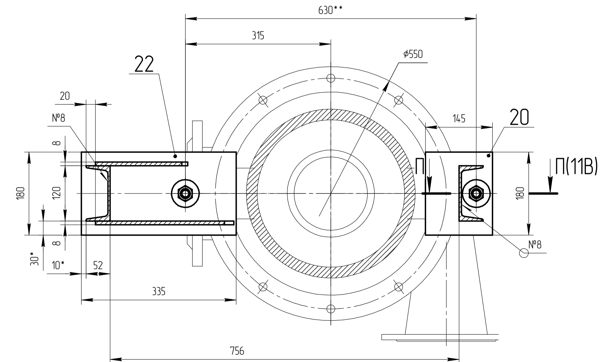
Д-Д(1:5)(7В)
