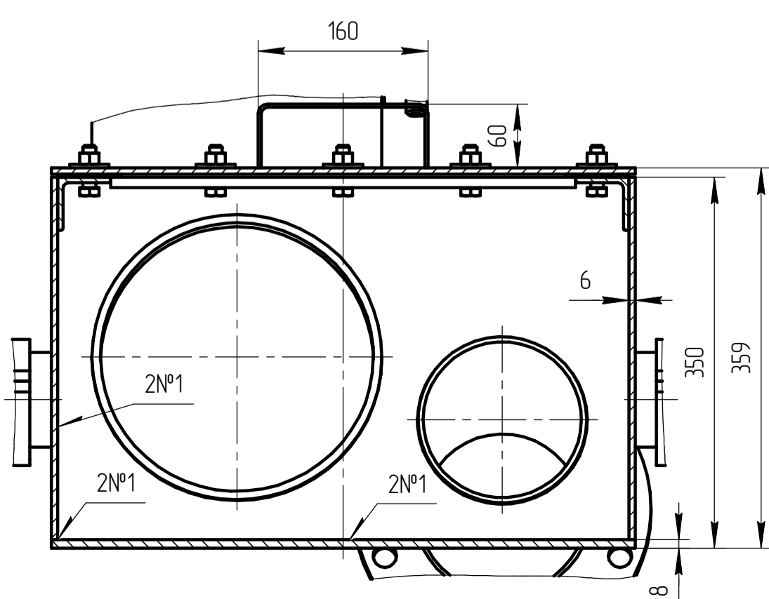
Р-Р(1:5)(5А)
